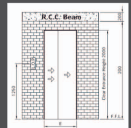
Telescopic Auto Door
